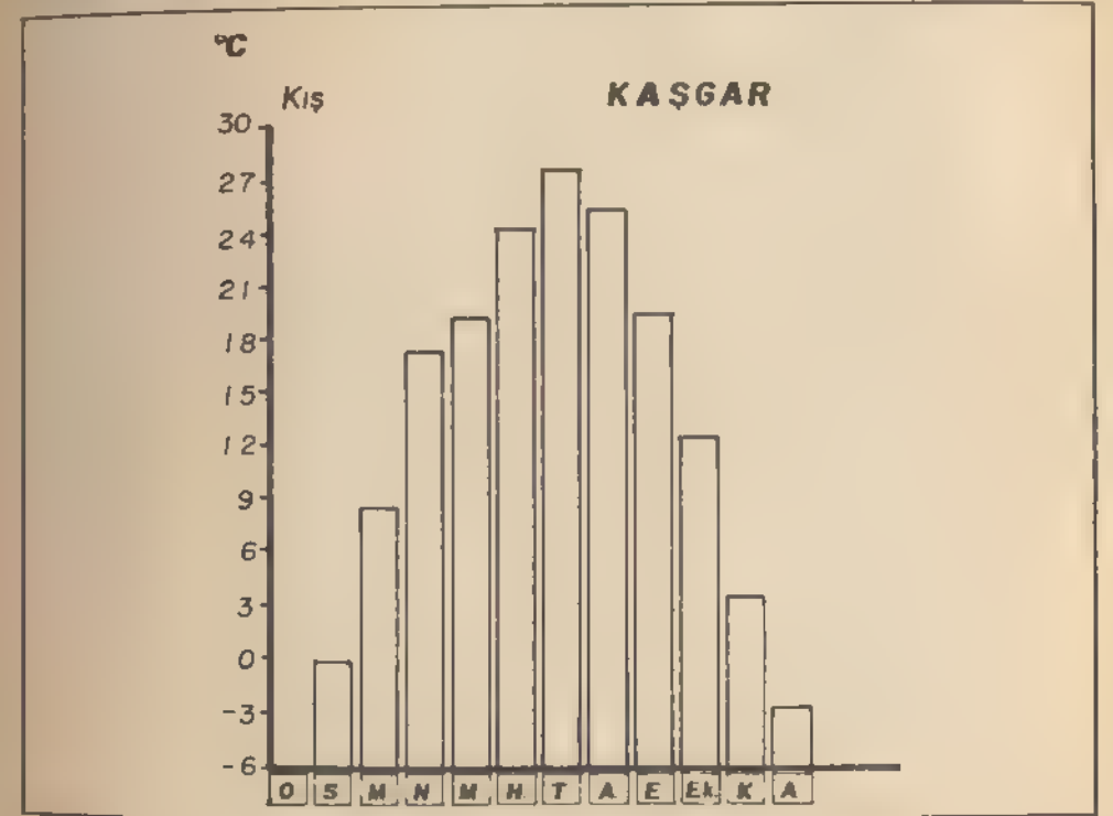
Şekil 3 - Kaşgar'ın sıcaklık rejimi
